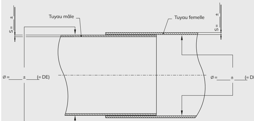
Figure 3 Information requise pour sélectionner le collier AccuSeal adapté
