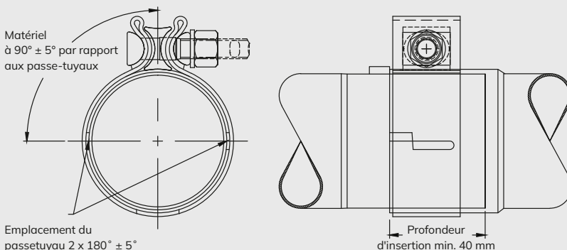
Figure 2 Exemple de tuyau d'échappement – Configuration de montage AccuSeal
